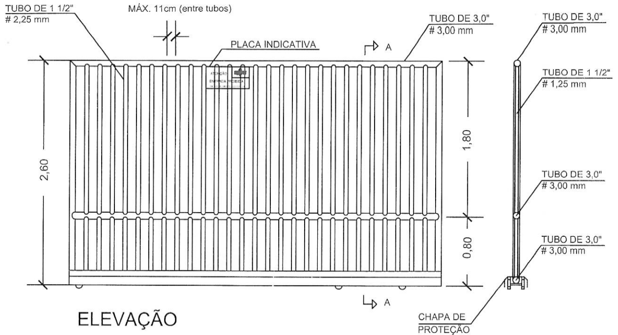
PORTÃO DE CORRER ETE
