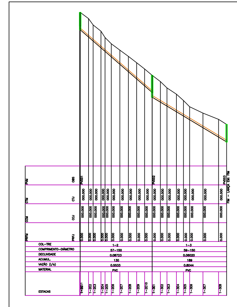
PERFIL DE REDE esc SEM
